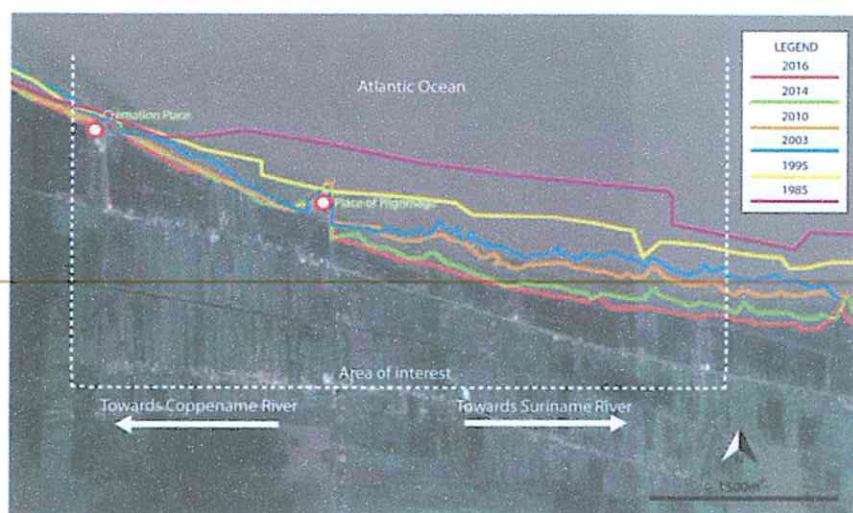
Figuur IV.1.1.1: Overzicht van het verloop van de kusterosie, periode 1985-2016
